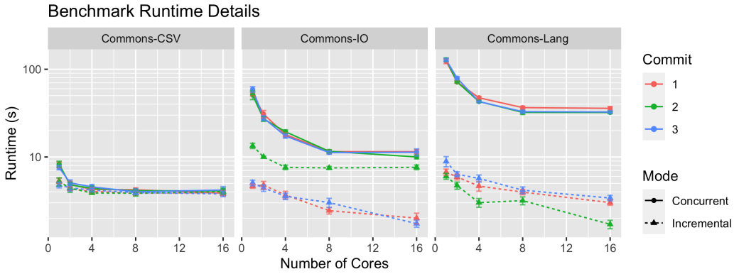
Fig. 30. Absolute runtimes of Apache Commons benchmarks
